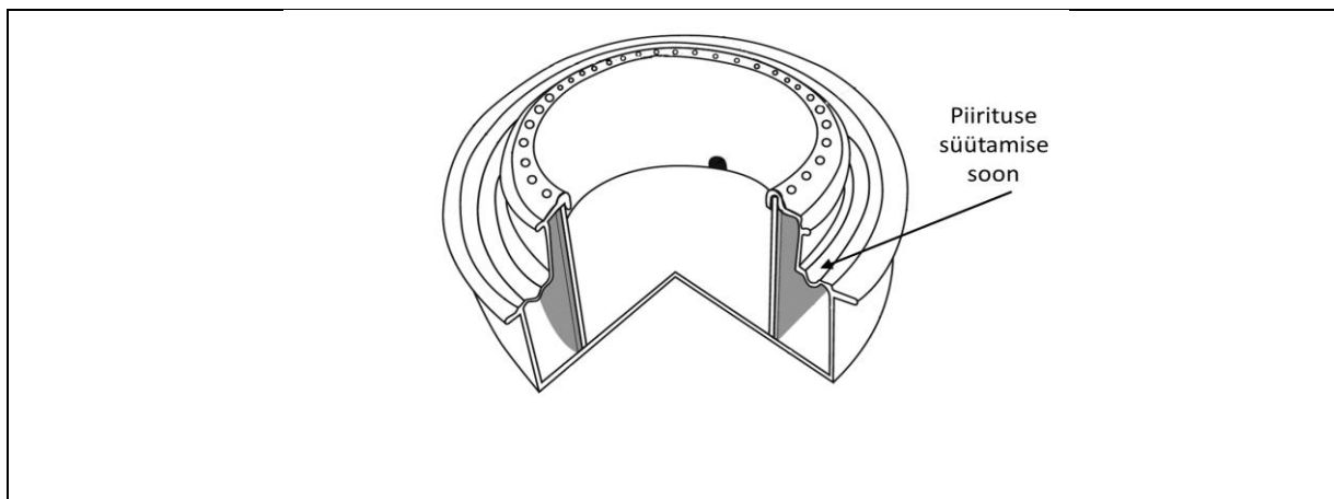
Joonis 1: Piirituspõleti läbilõige
